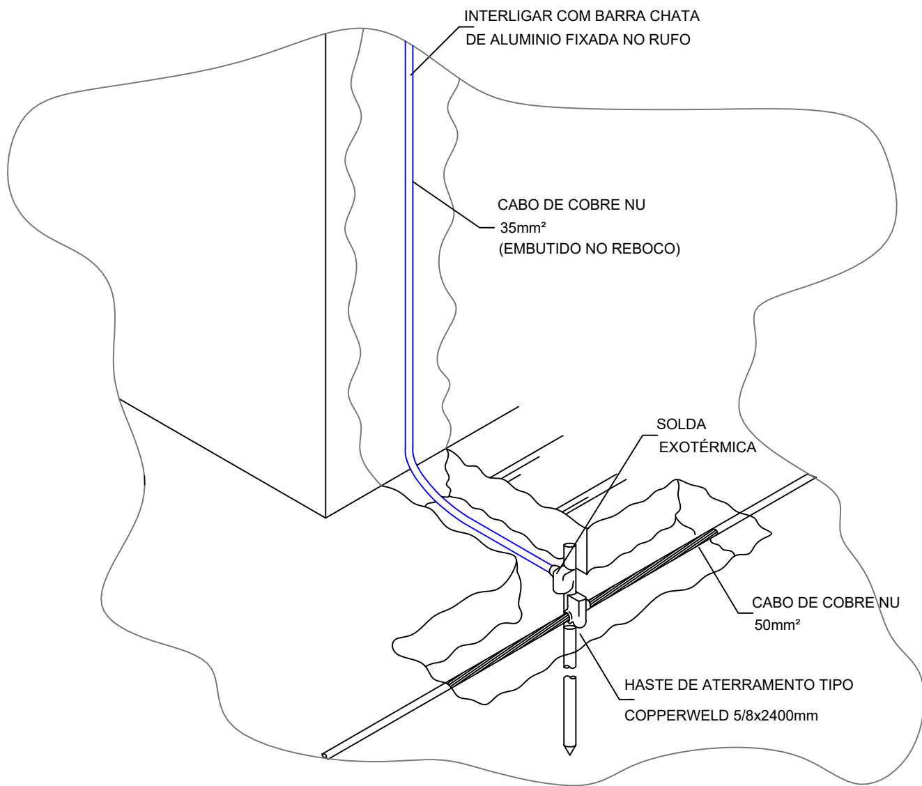
DETALHE 3 DESCIDA EMBUTIDA NA ALVENARIA S/ ESCALA
