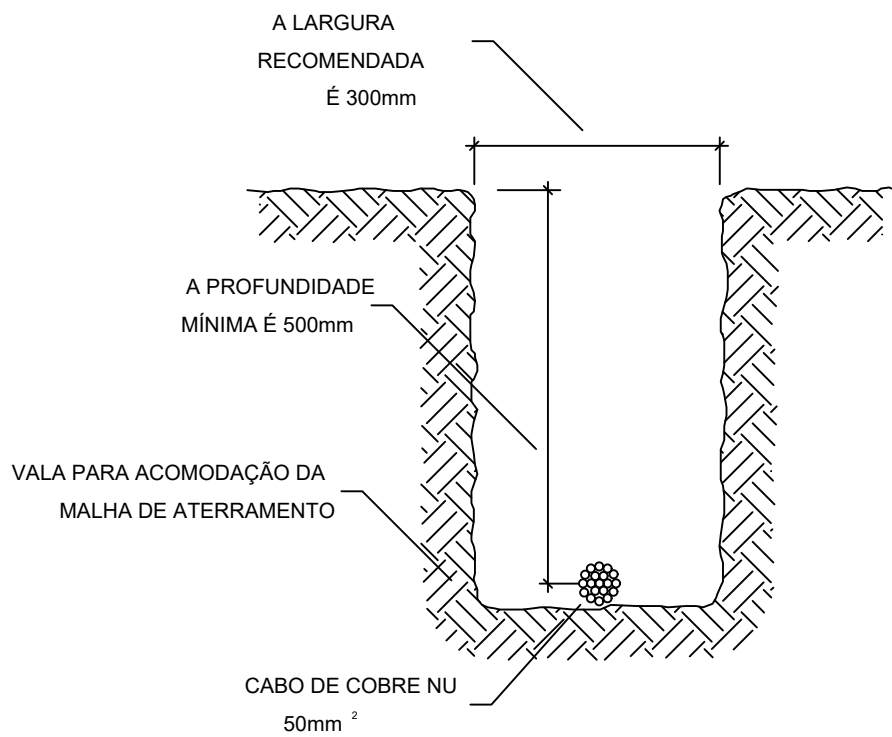
DETALHE 1 VALA DE ATERramento S/ ESCALA
