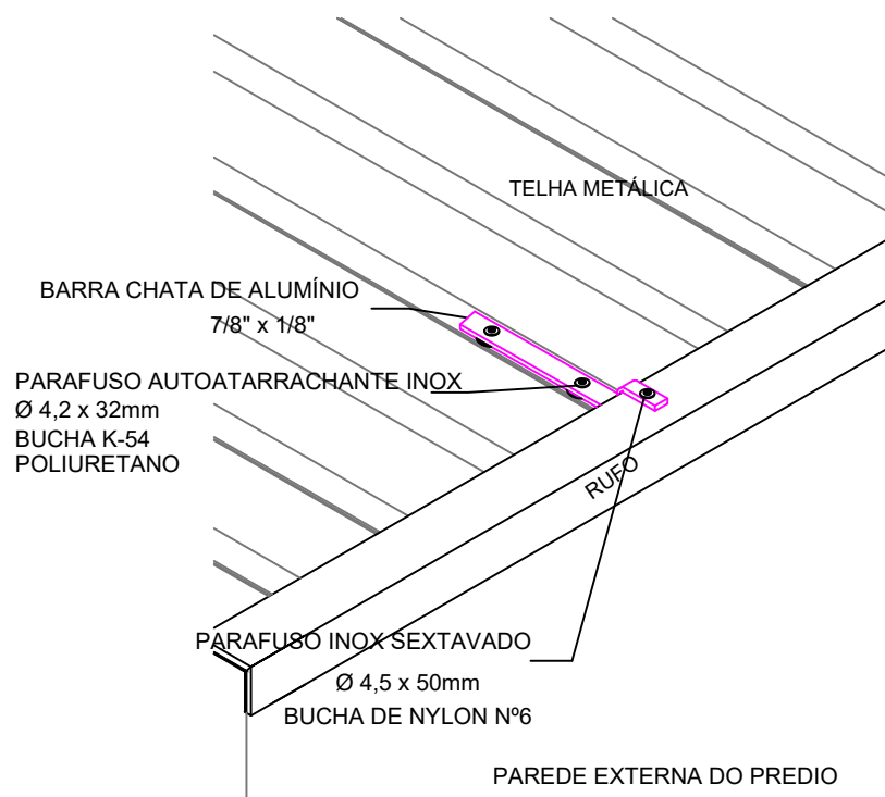
DETALHE 4 INTERLIGAÇÃO TELHADO COM RUFO S/ ESCALA
