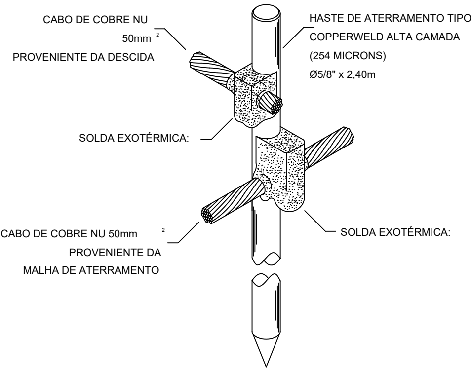
DETALHE 2 SOLDA EXOTÉRMICA S/ ESCALA
