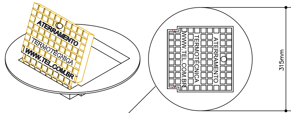
CAIXA DE INSPEÇÃO TIPO SOLO EM PVC COM TAMPA DE FERRO FUNDIDO REFORÇADA COM BOCAL INTERIOR QUADRADO ARTICULADO E BORDA EXTERIOR REDONDA Ø300mm
