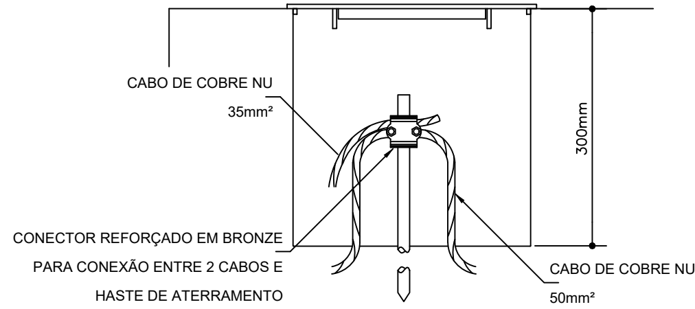
DETALHE 5 CAIXA DE INSPEÇÃO DE SOLO S/ ESCALA
