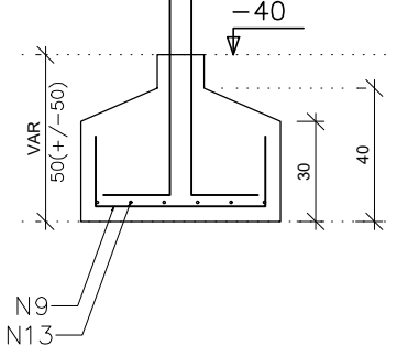
CORTE ESC 1:25
