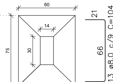
S3 PLANTA ESC 1:25
