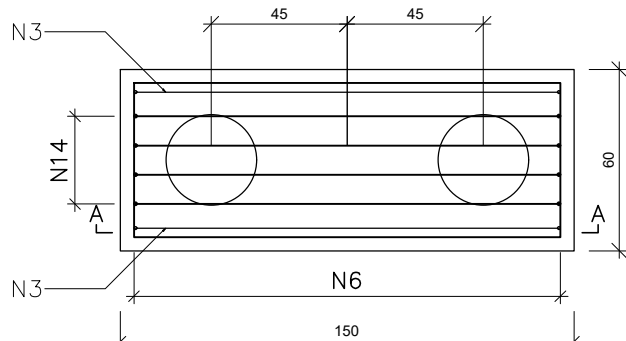
B6=B7 2xC25 PLANTA ESC 1:25
