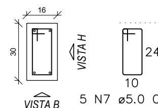
TERREO - L1 SEÇÃO ESC 1:20
