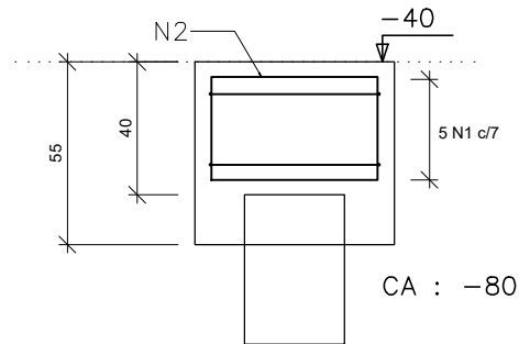
CORTE ESC 1:25
