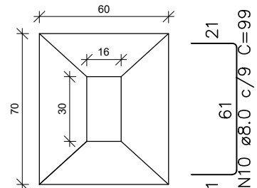
S1 PLANTA ESC 1:25
