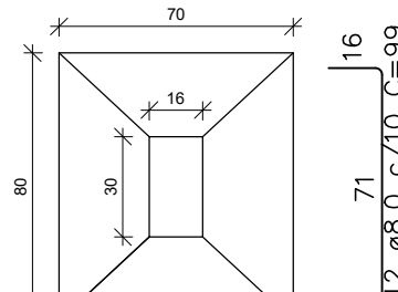
S2 PLANTA ESC 1:25
