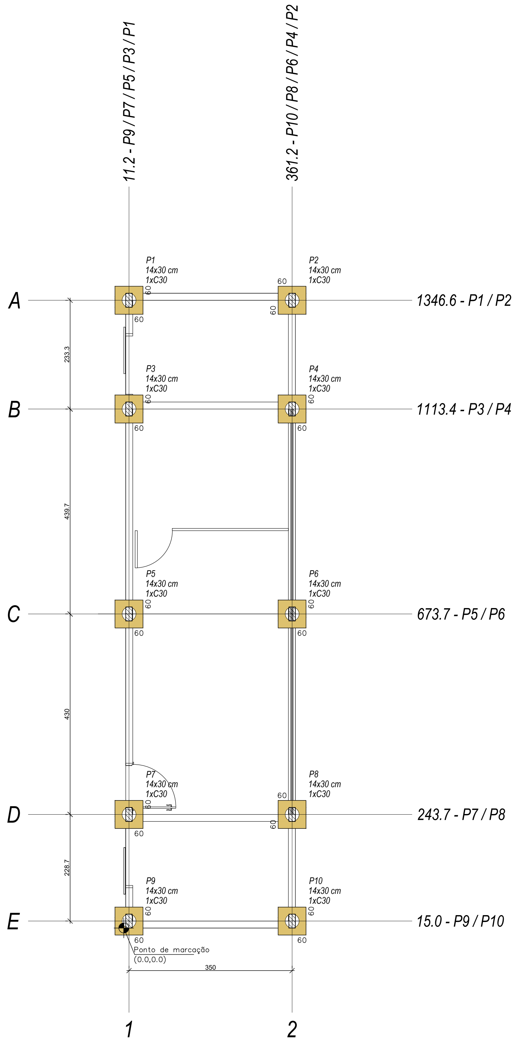
PLANTA DE LOCAÇÃO escala 1:50
