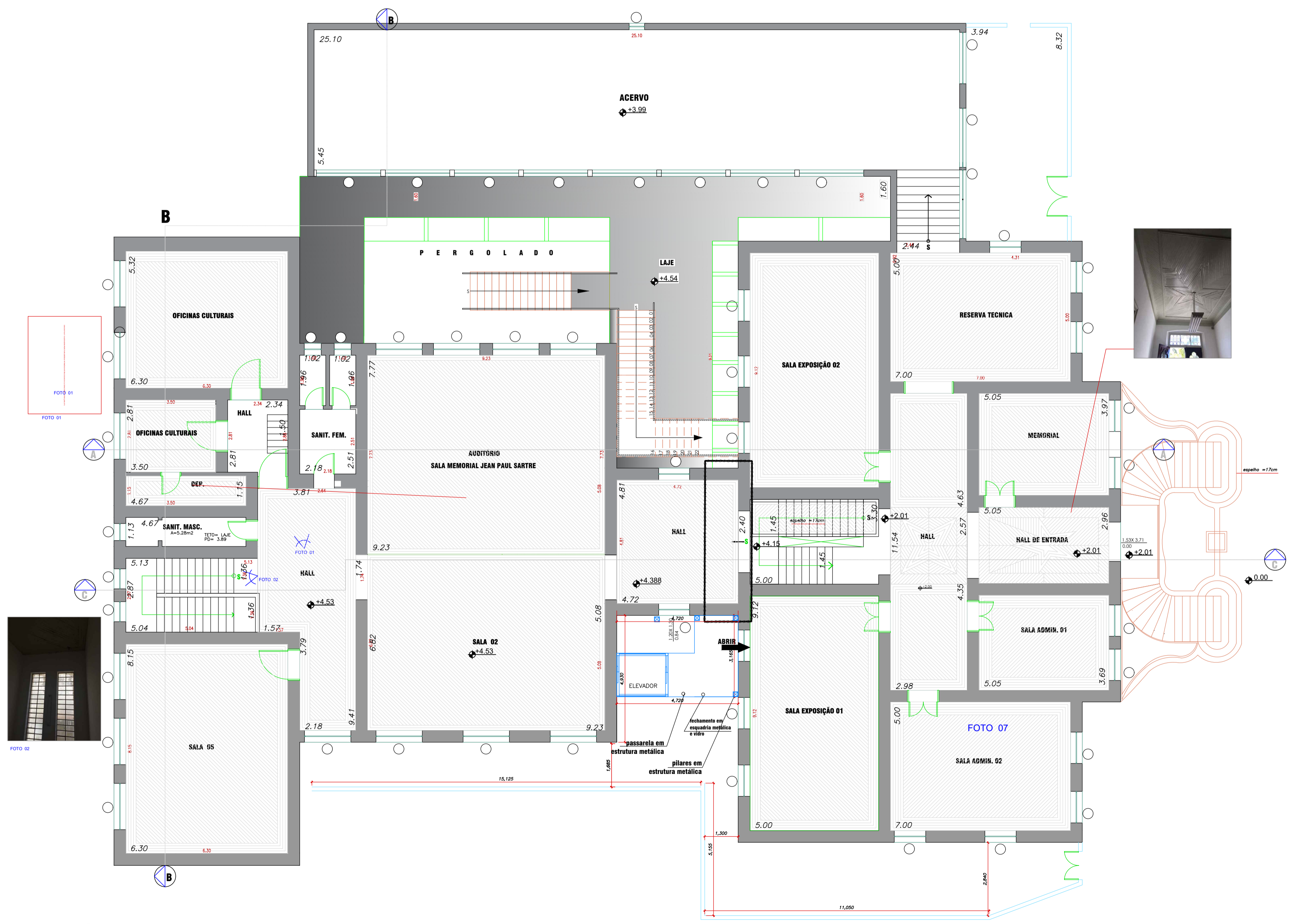
PLANTA-BAIXA: 1º PAVIMENTO - FORRO -EXISTENTE Escala 1:100
