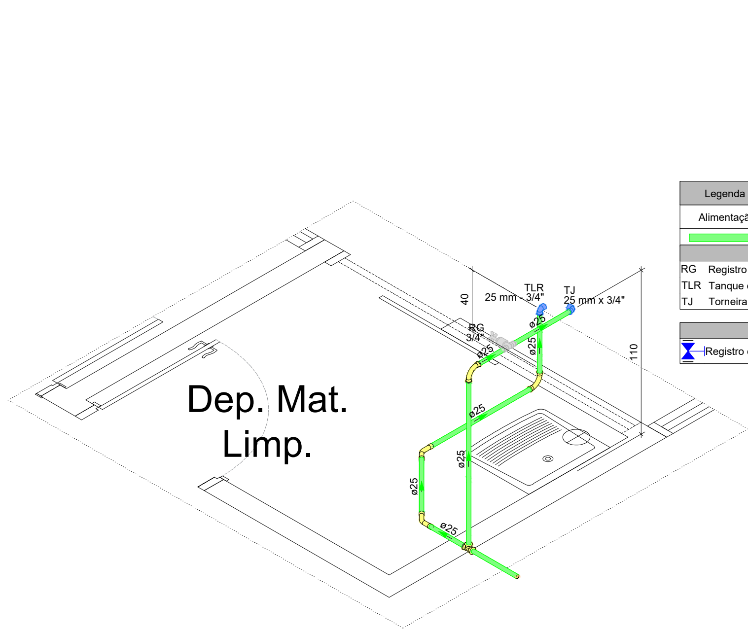
Detalhe HID-13 Escala 1:25
