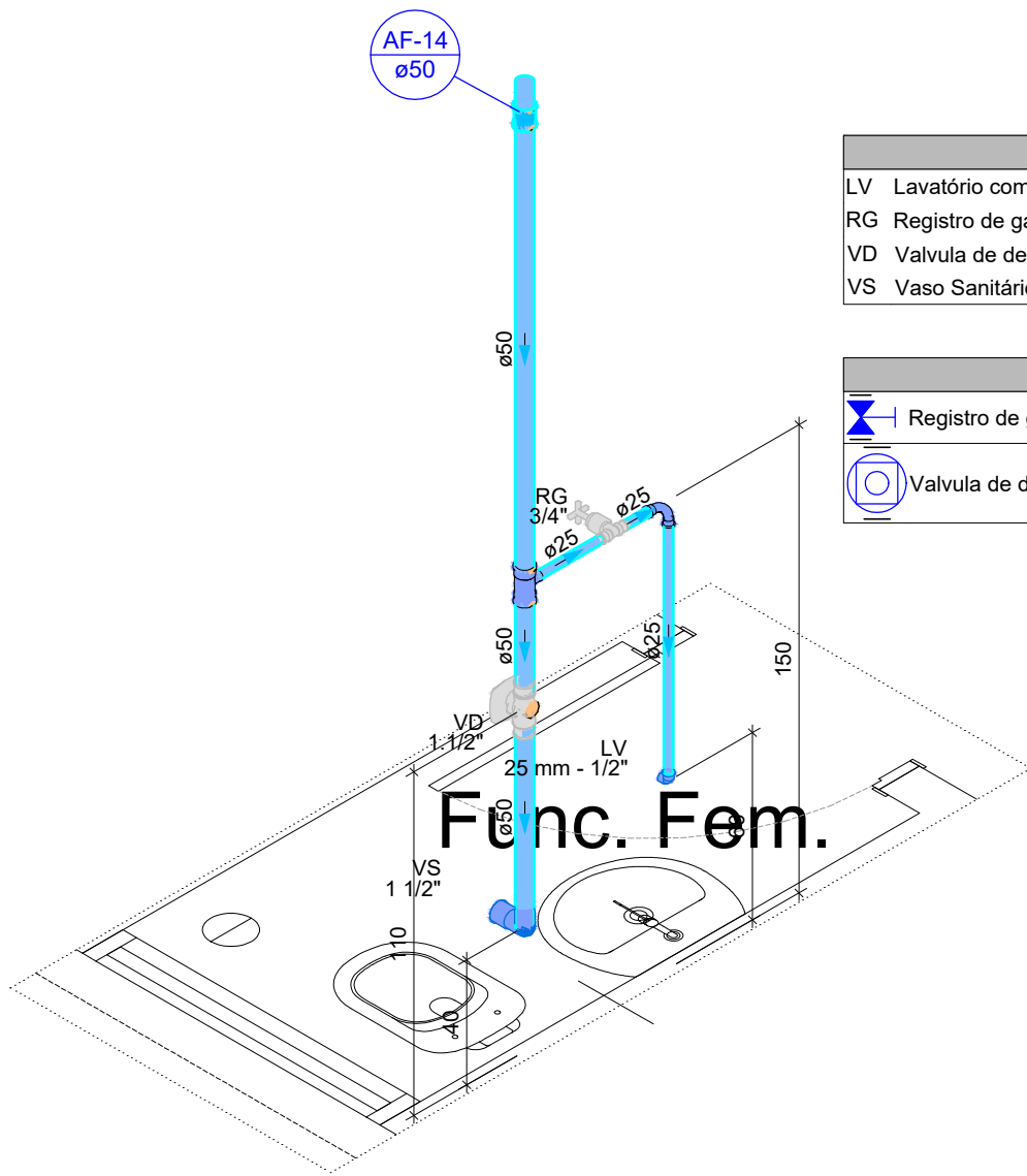
Detalhe HID-14 Escala 1:25
