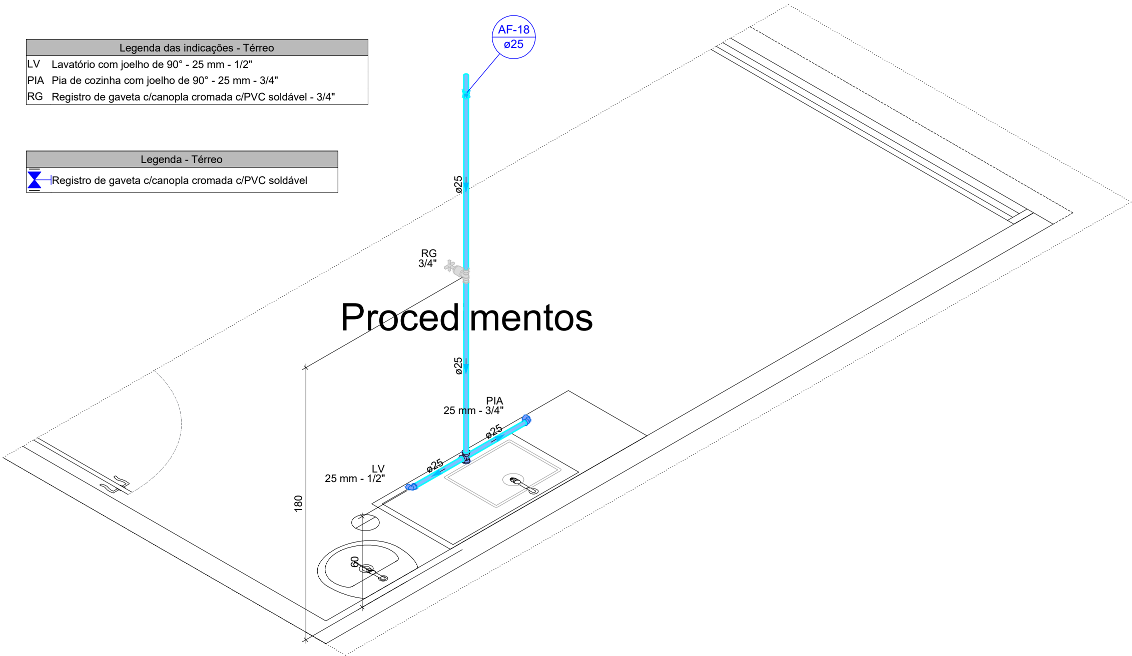
Detalhe HID-18 Escala 1:25
