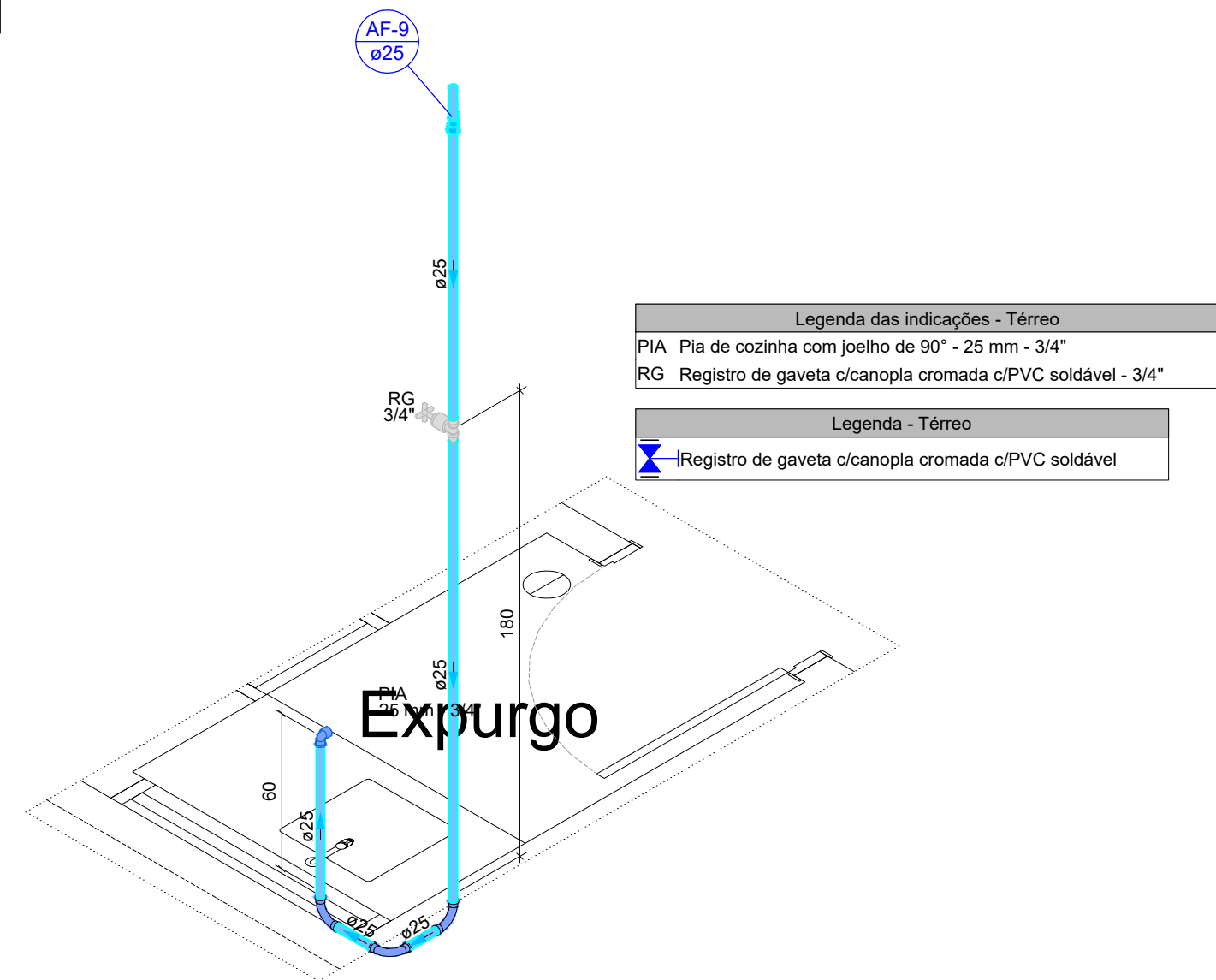
Detalhe HID-9 Escala 1:25
