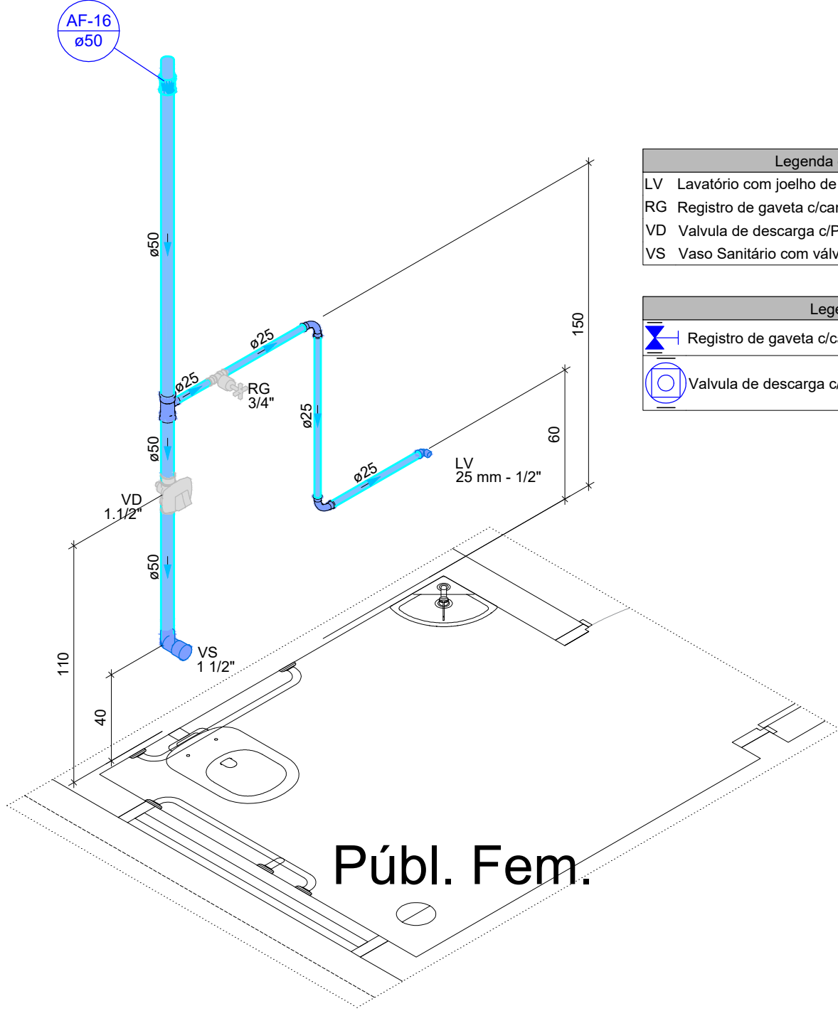
Detalhe HID-16 Escala 1:25
