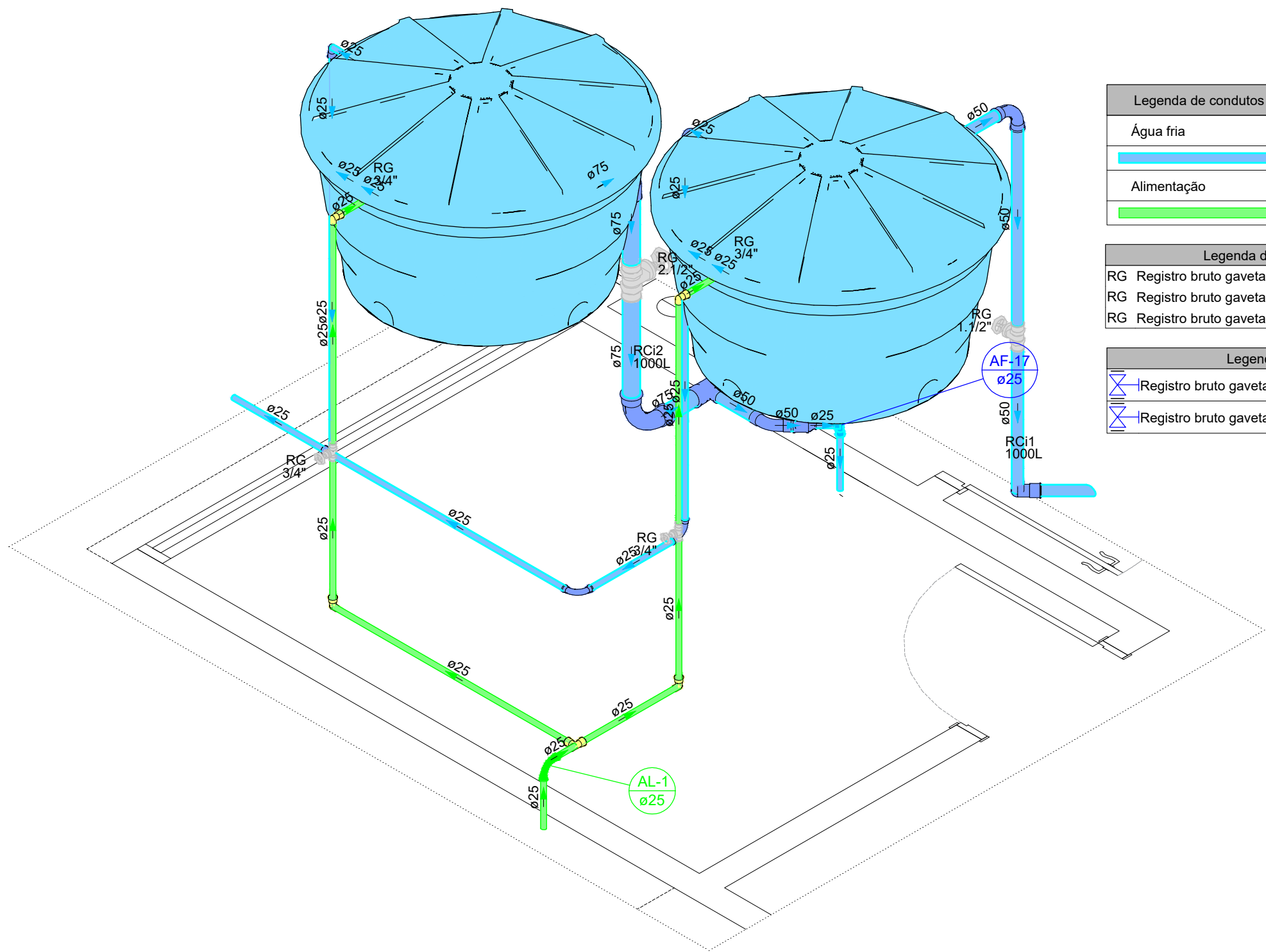
Detalhe HID-19 Escala 1:25
