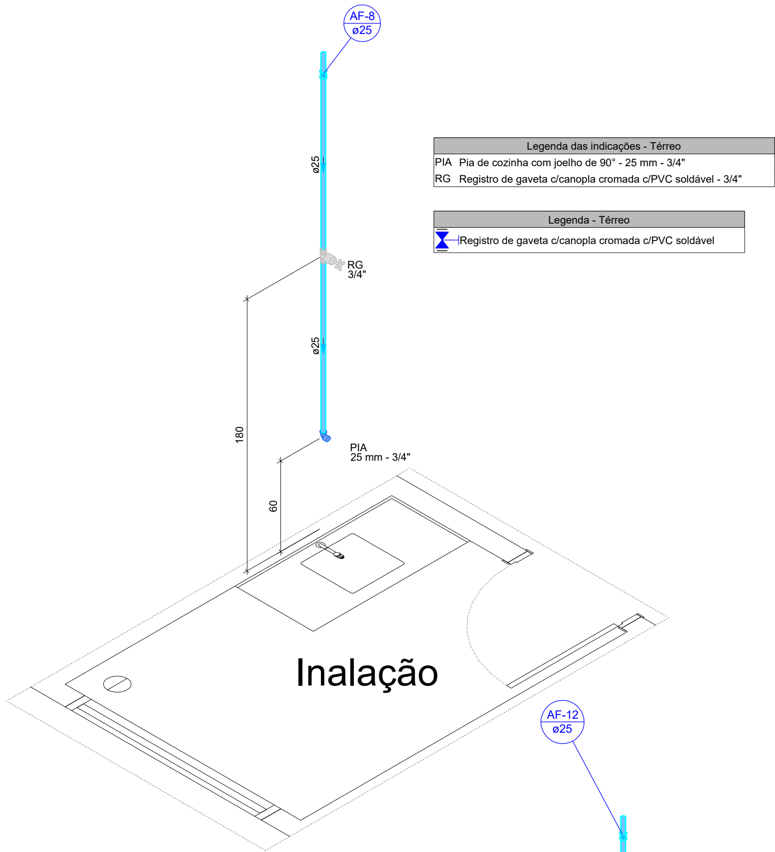
Detalhe HID-8 Escala 1:25
