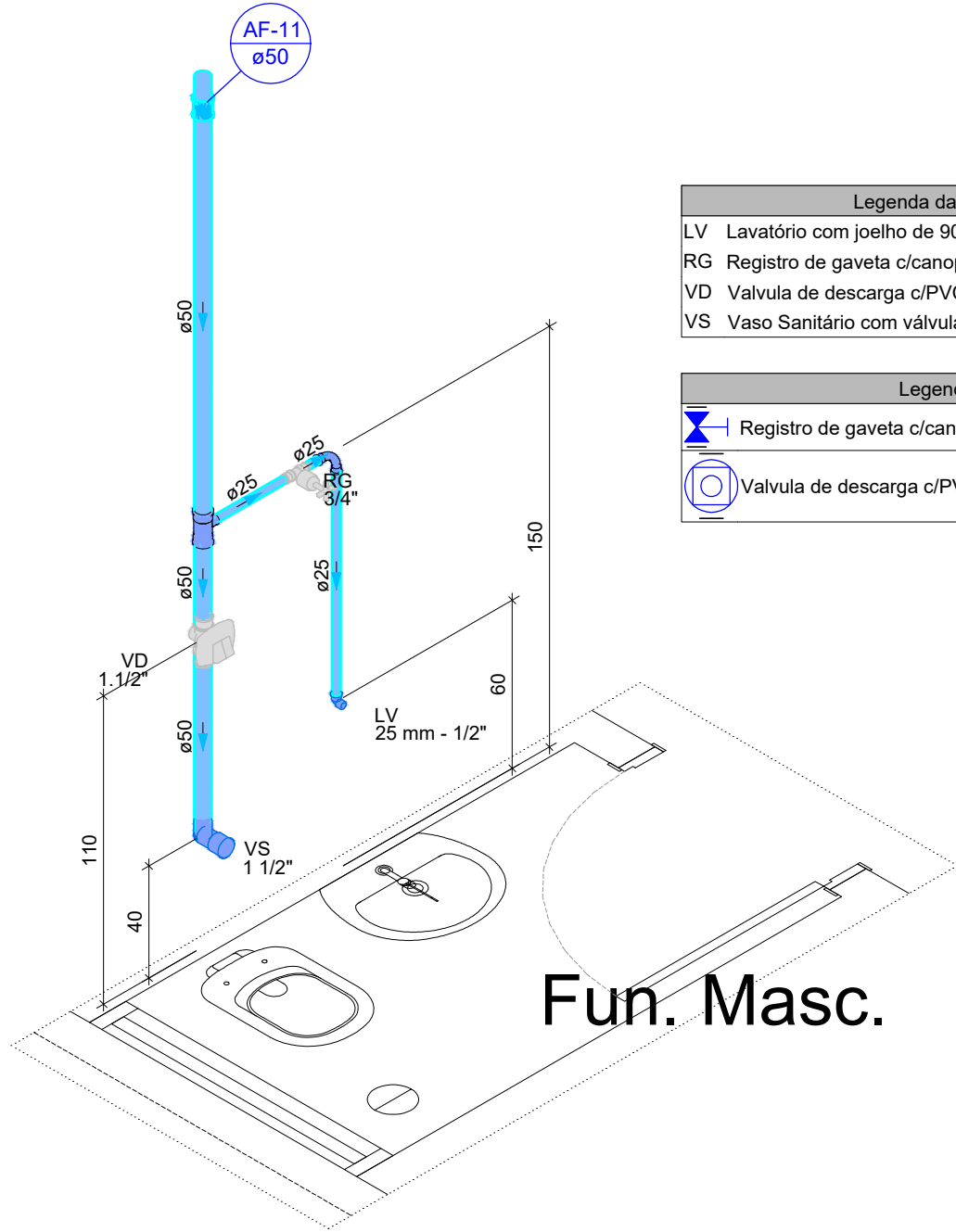
Detalhe HID-11 Escala 1:25
