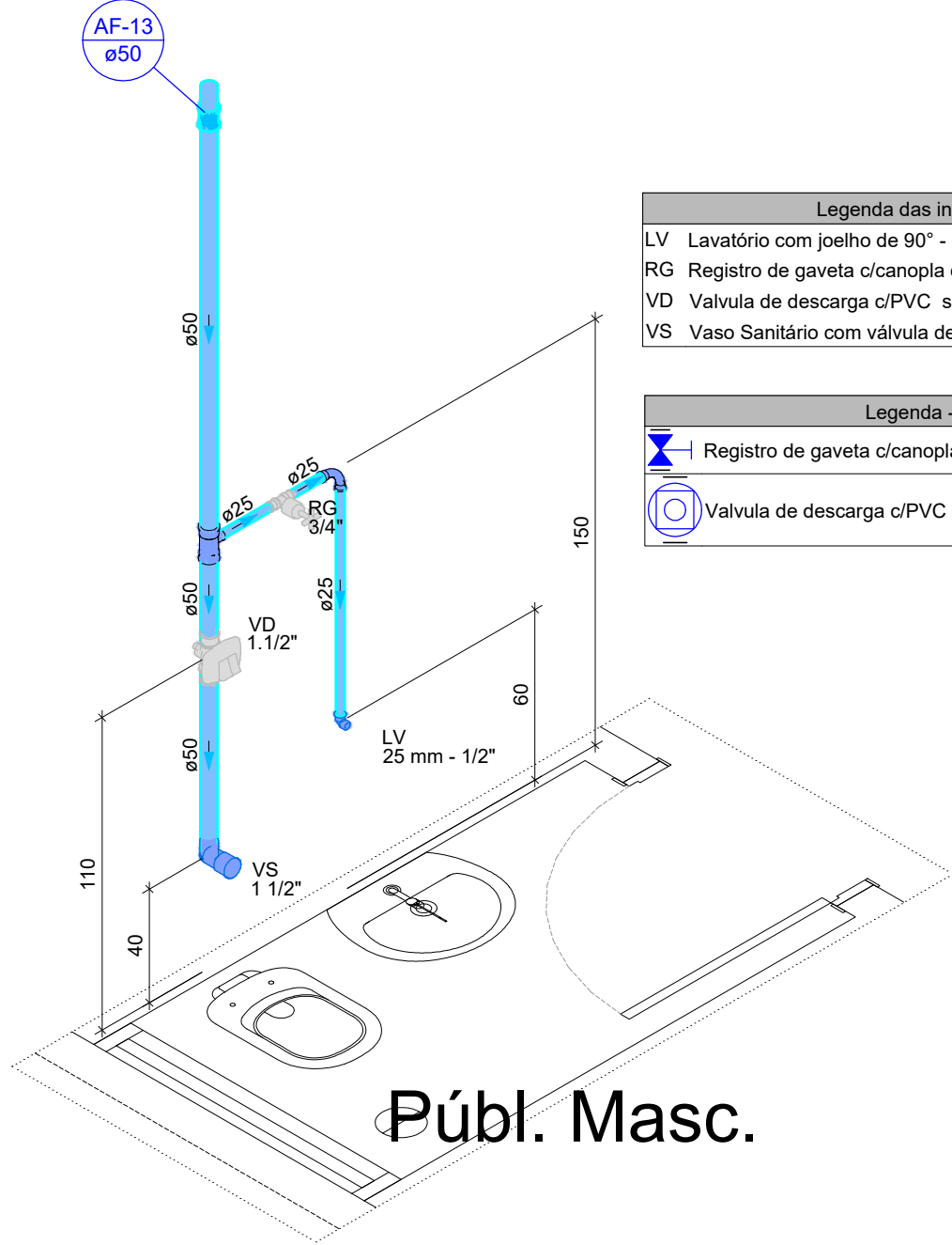
Detalhe HID-15 Escala 1:25
