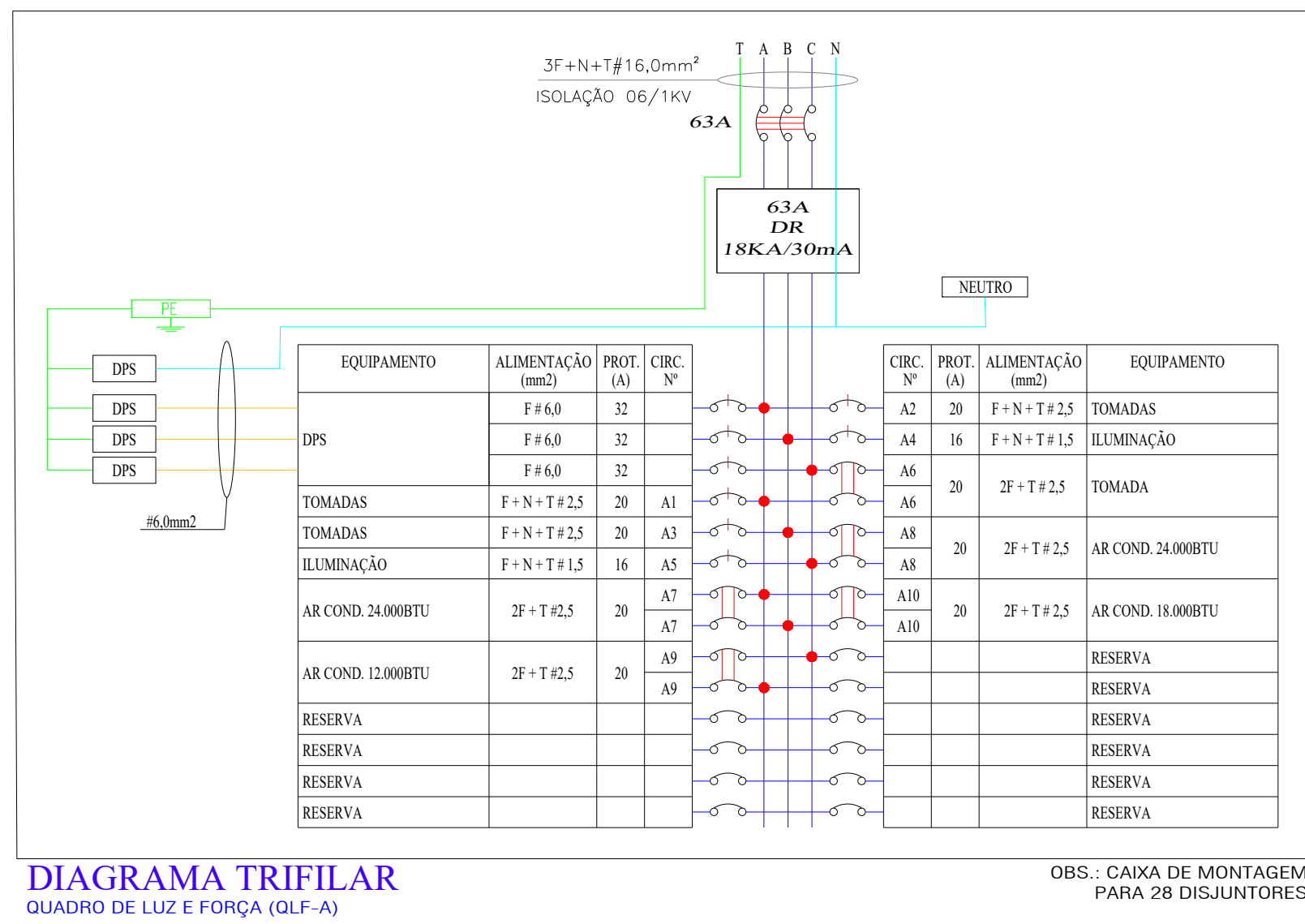
DIAGRAMA TRIFILAR QUADRO DE LUZ E FORÇA (OLF-A)
