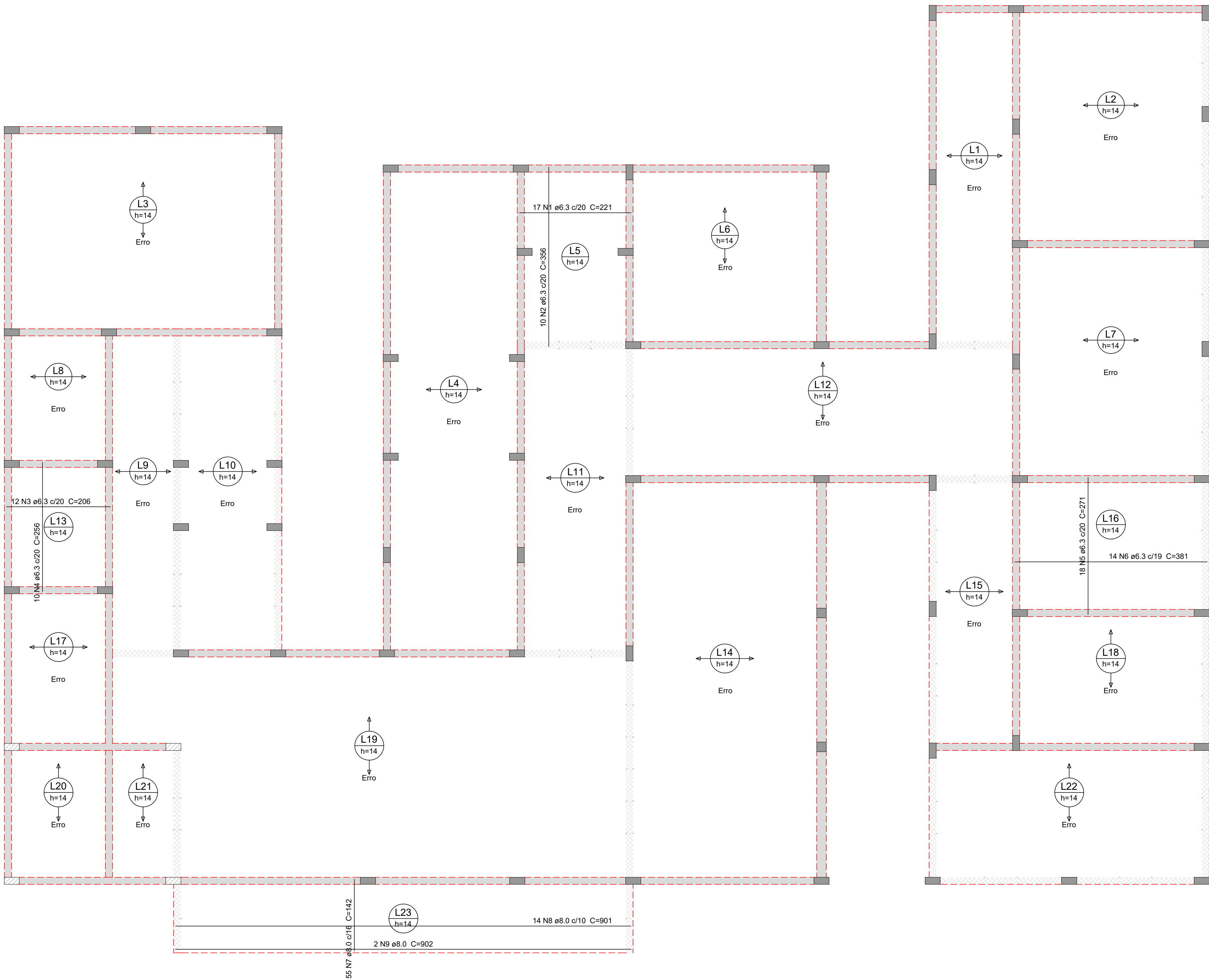
Armação positiva das lajes do pavimento Térreo
