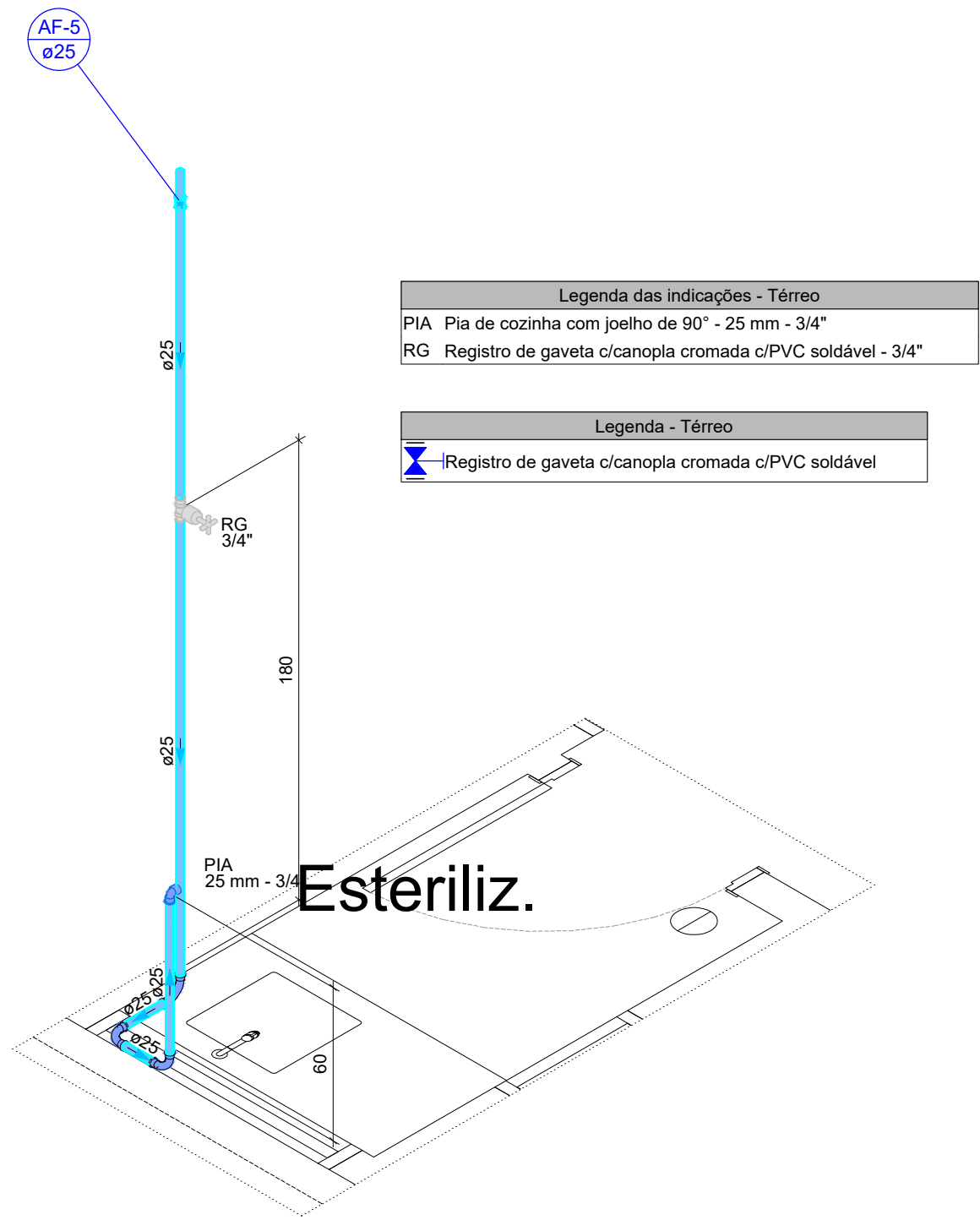
Detalhe HID-7 Escala 1:25
