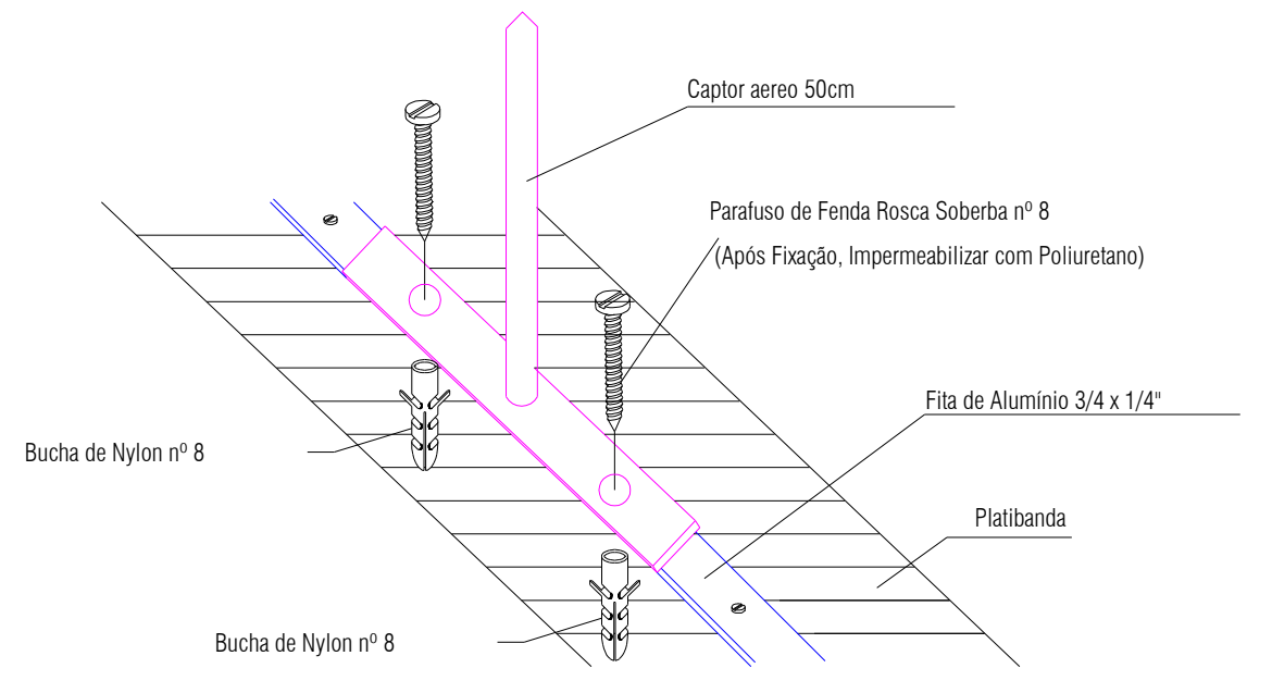
DETALHE DA FIXAÇÃO DO CAPTOR
