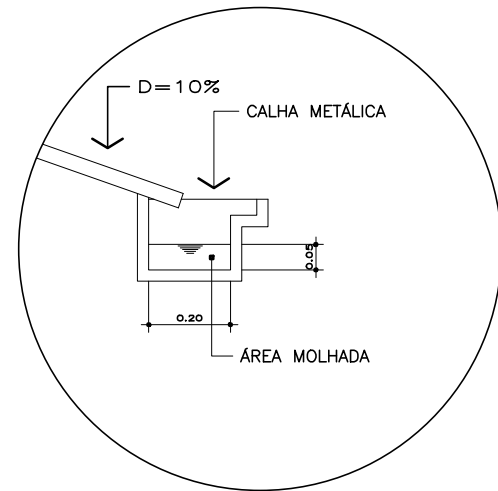
DET. CALHA
