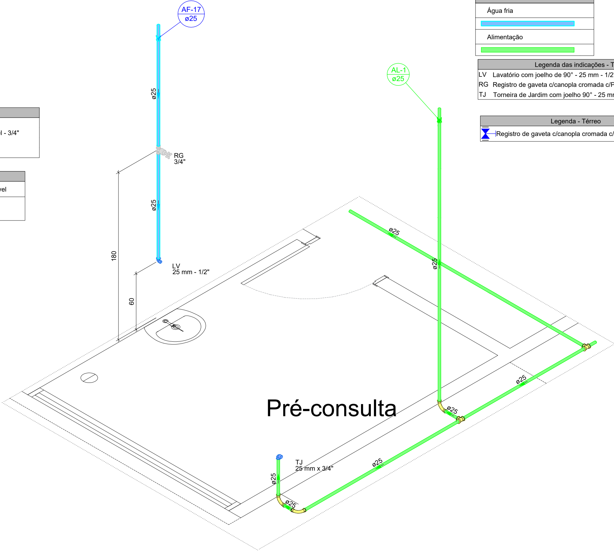
Detalhe HID-17 Escala 1:25
