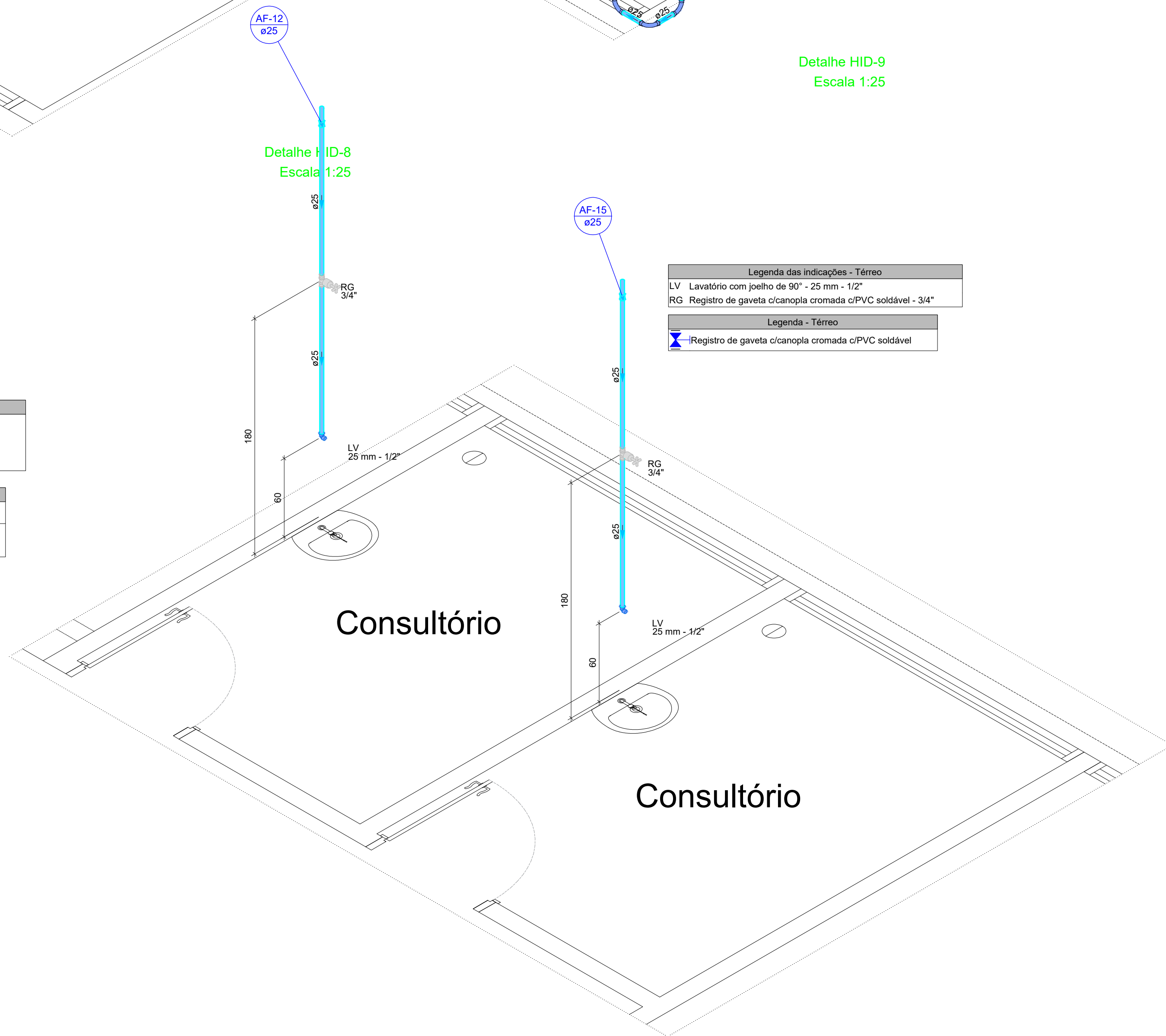
Detalhe HID-12 Escala 1:25
