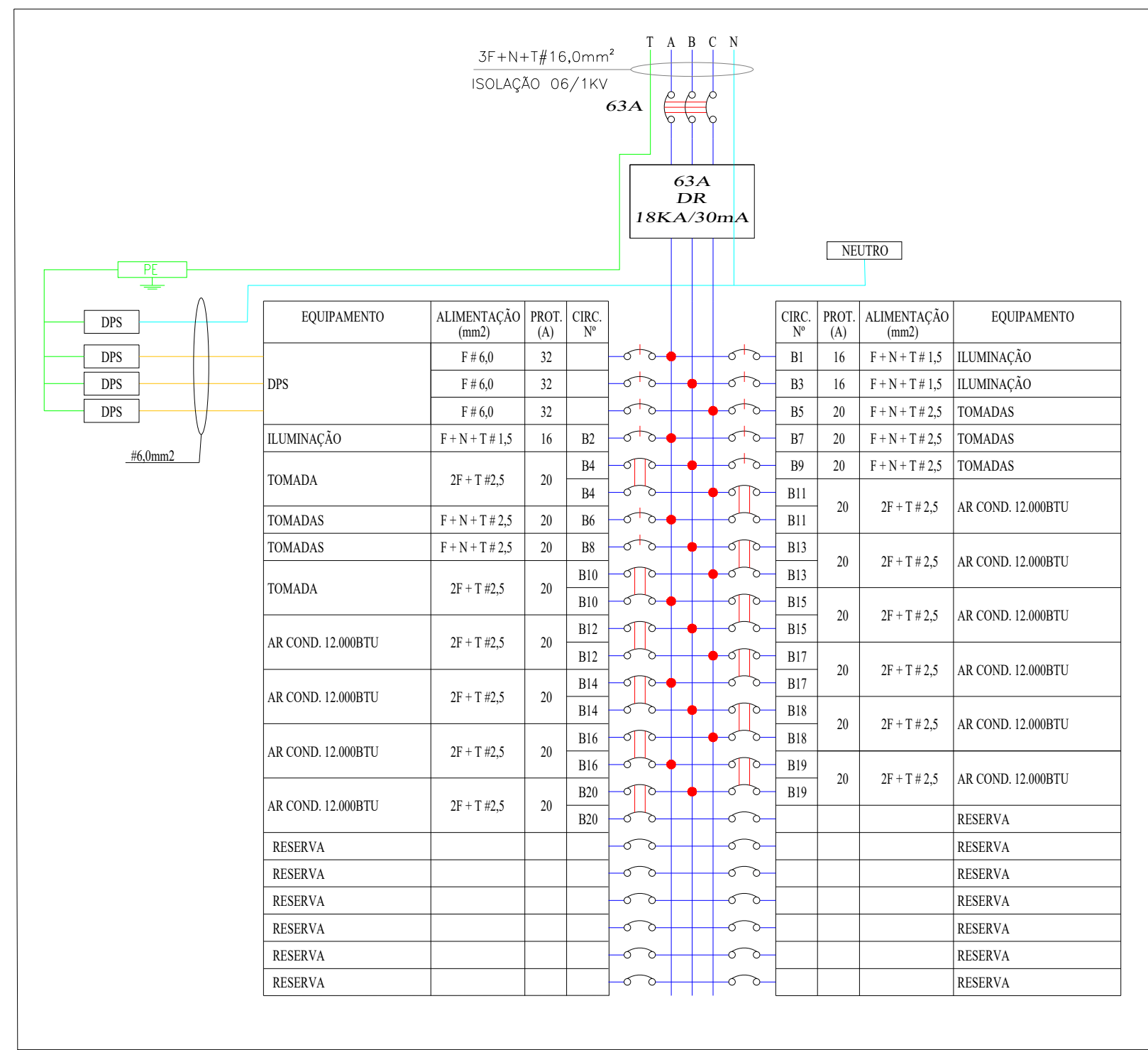
DIAGRAMA TRIFILAR QUADRO DE LUZ E FORÇA (OLF-B)
