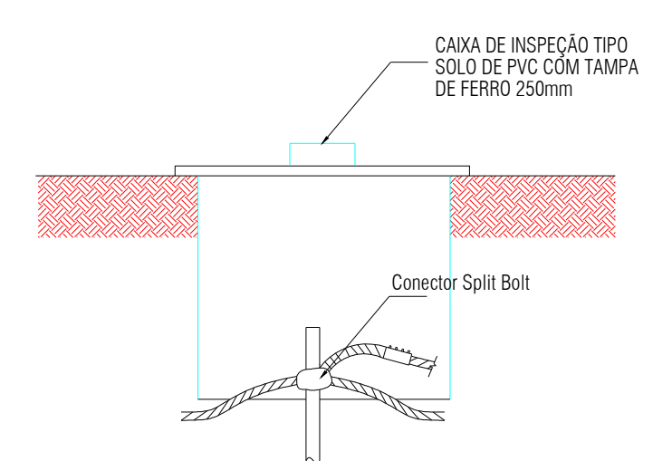
HASTE EM CAIXA DE INSPEÇÃO TIPO SOLO
