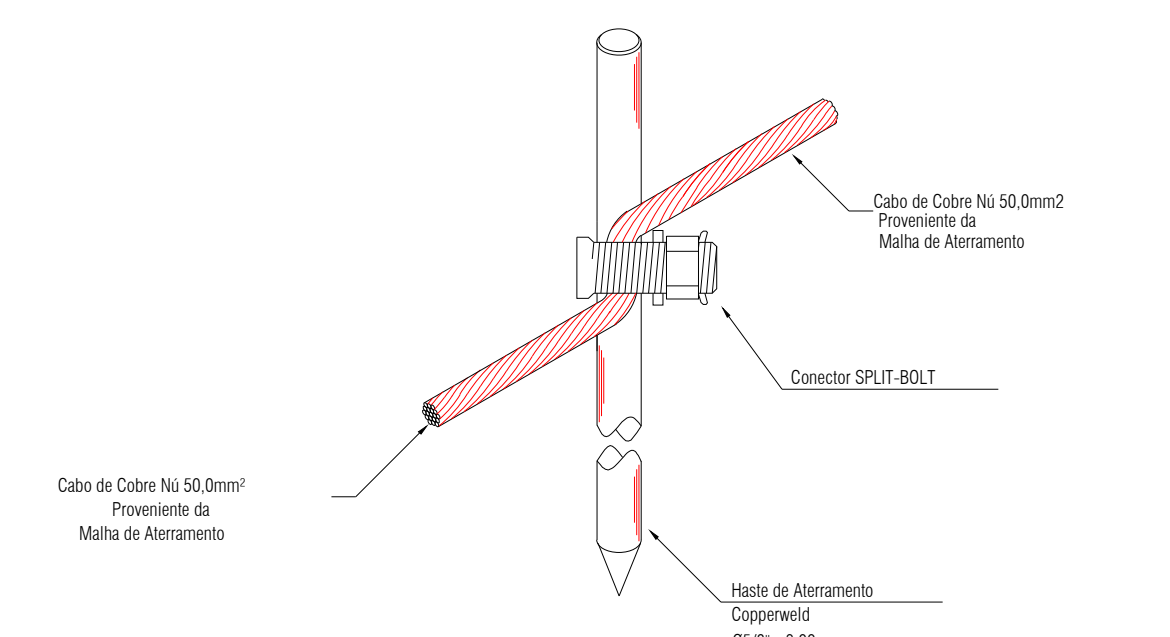
DETALHE DE CONEXÃO DO CABO DE COBRE PROVENIENTE DO ANEL INFERIOR À HASTE DE ATERRAMENTO
