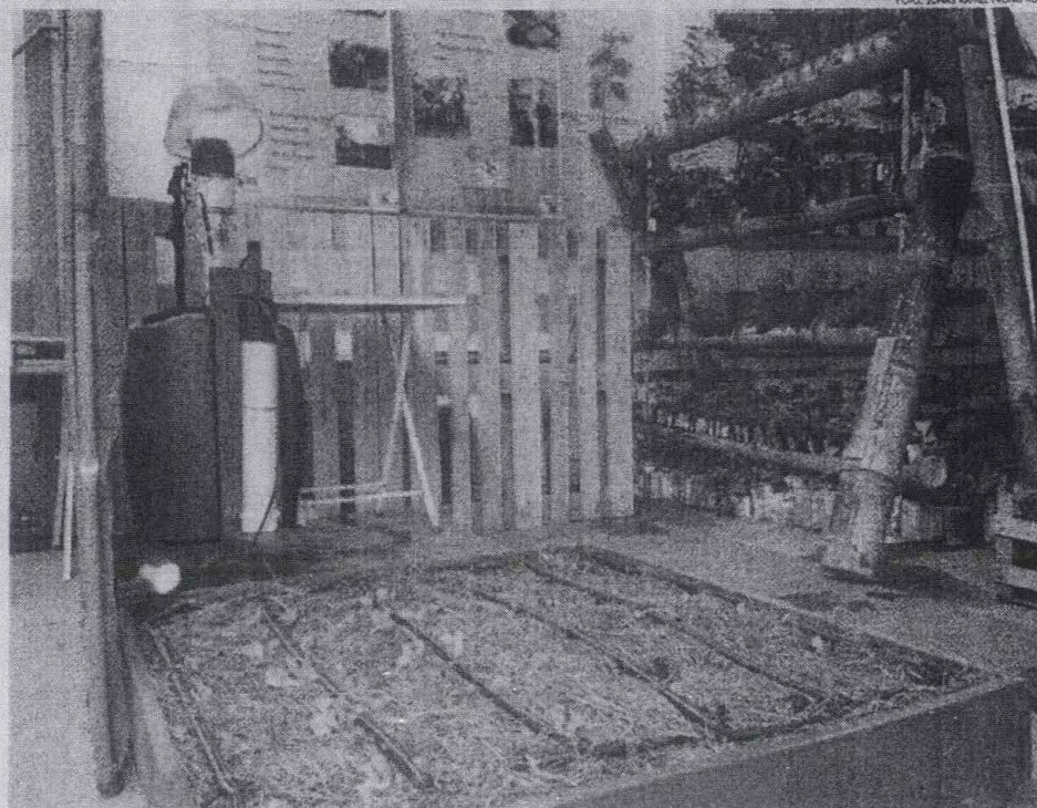
Irrigador movido a energia solar produzido por alunos de Engenharia Agrônômica da Uniara
